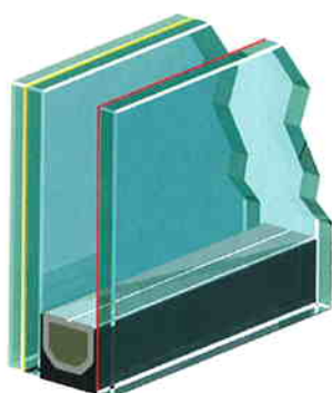
Vitrage anti-vandalisme SP510 SP510 / 16 argon / 4 ITR
