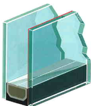
Vitrage à faible émissivité 4/16 argon / 4 ITR
