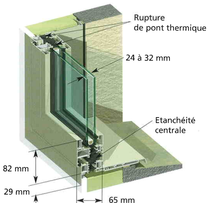
Ouvrant Apparent
