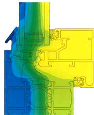
Courbes isothermiques
